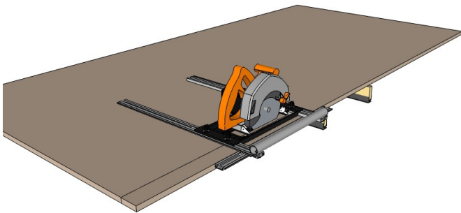
Using the Universal Edge Guide*
